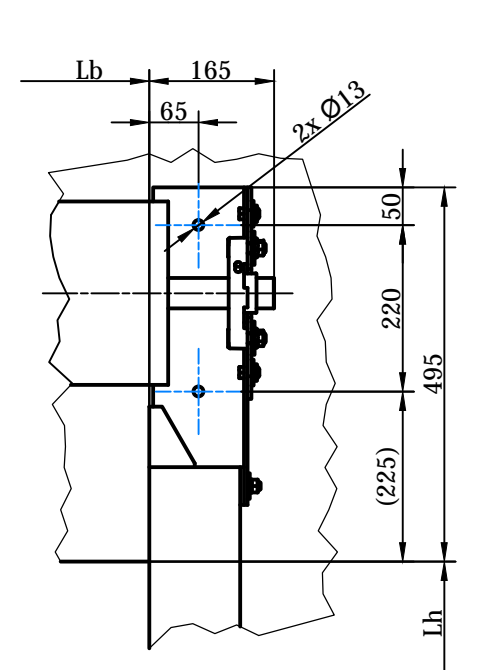
Det. D ( 1 : 10 )
