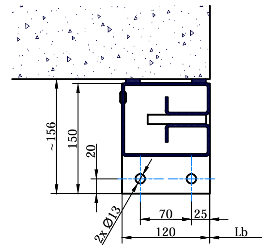
A-A ( 1:5 )
