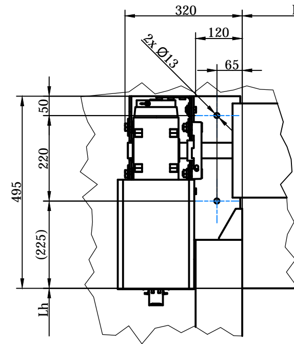
Det. C ( 1 : 10 )
