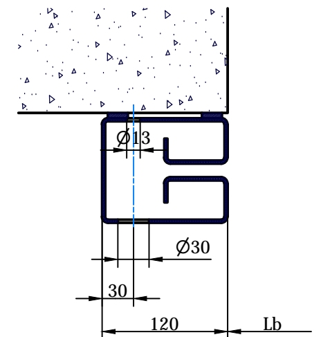
B-B ( 1:5 )
